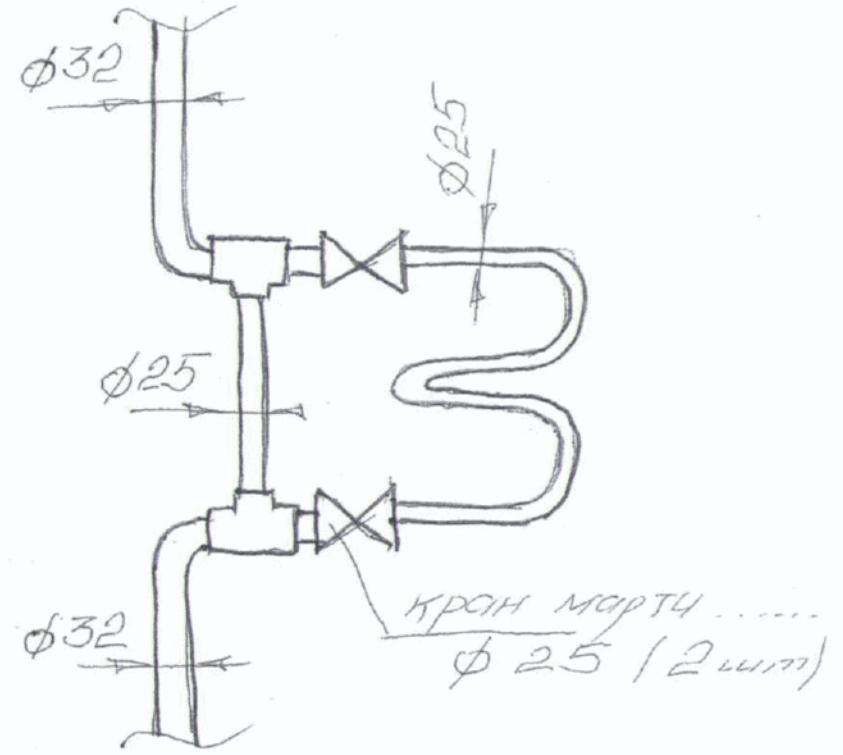
Схема ГВС после переустройства
