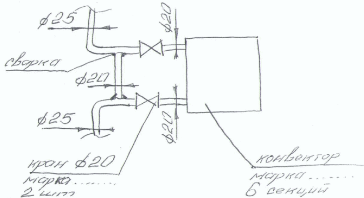
Схема ЦО после переустройства Комната 16 м 2
